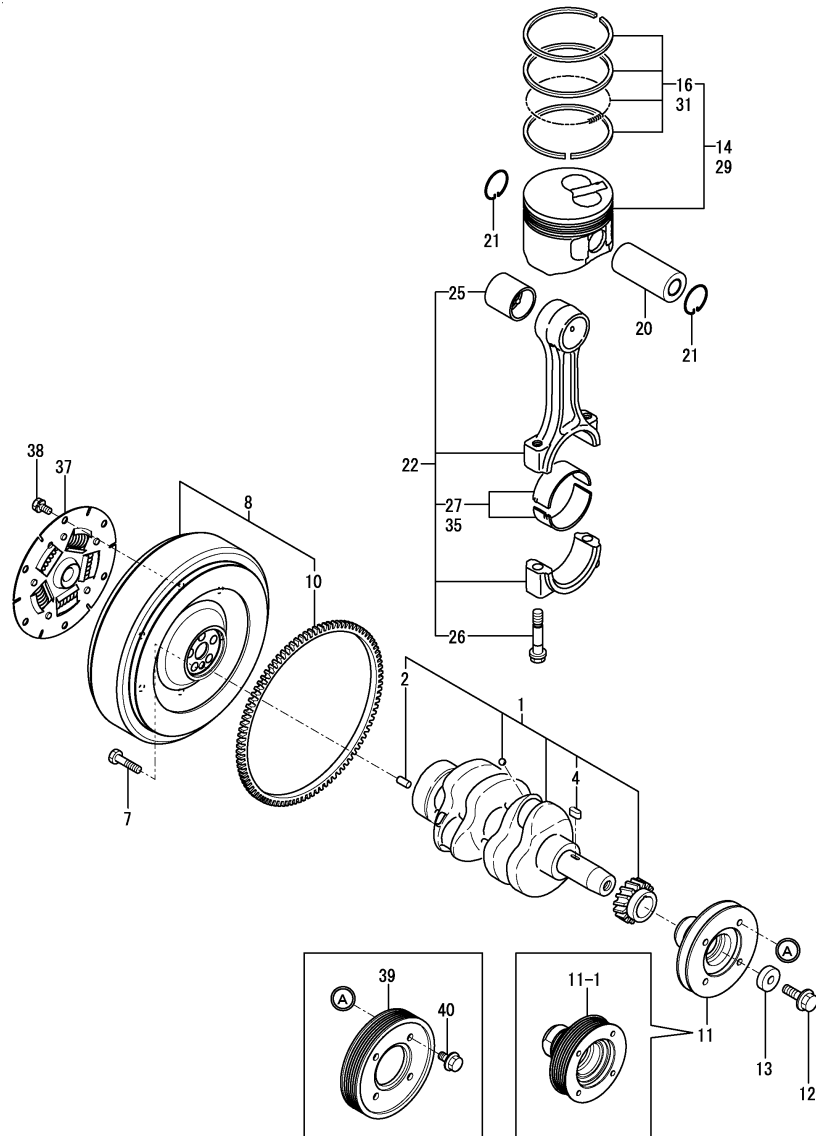
Fig.10. CRANKSHAFT & PISTON
